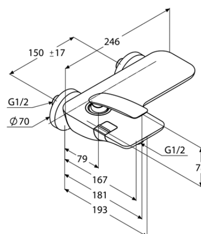
Размеры
